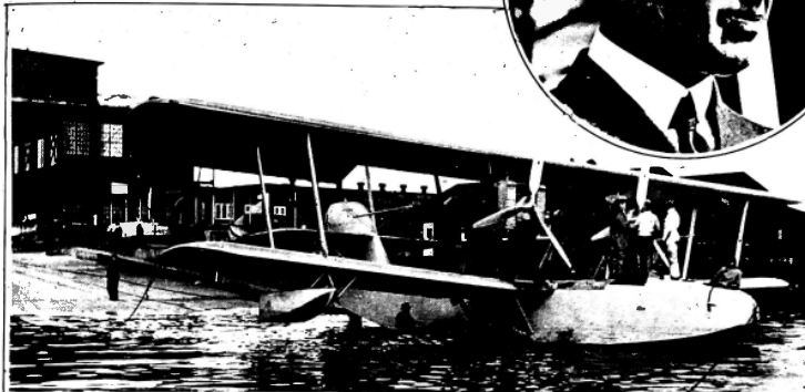
El PN-10 N° 1, el gran hidroplano norteamericano que intentaba realizar sin escalas el vuelo Hampton Roads-Panamá, y se vio obligado a acuatizar a 213 millas al sur de la isla de Pinos por roturas en el motor. En el círculo: el Comandante BARTLETT, que condujo el PN-10 N° 2, y que por falta de combustible aterrizó en Nueva Gerona, después de recorrer 1896 kilómetros en catorce horas y veinte minutos, y prosiguió el emprendido vuelo.
